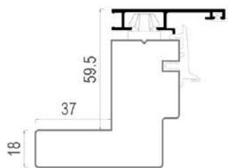
Battuta 37 mm
