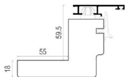
Battuta 55 mm
