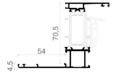
Battuta 54 mm
