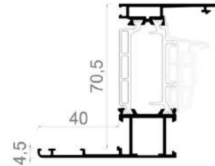
Battuta 40 mm
