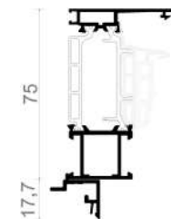
Telaio rasomuro
