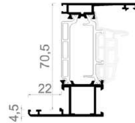
Battuta 22 mm
